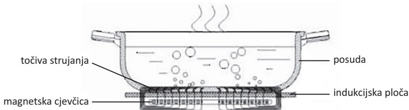
Shema grijanja
