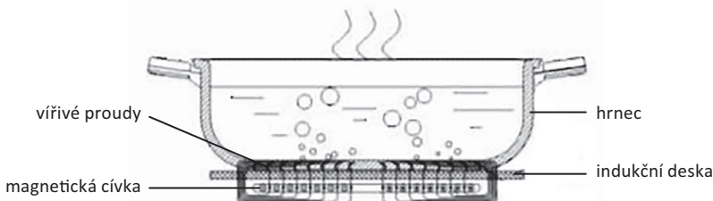
Schéma ohřevu
