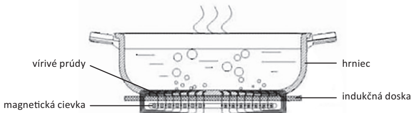
Schéma ohrevu
